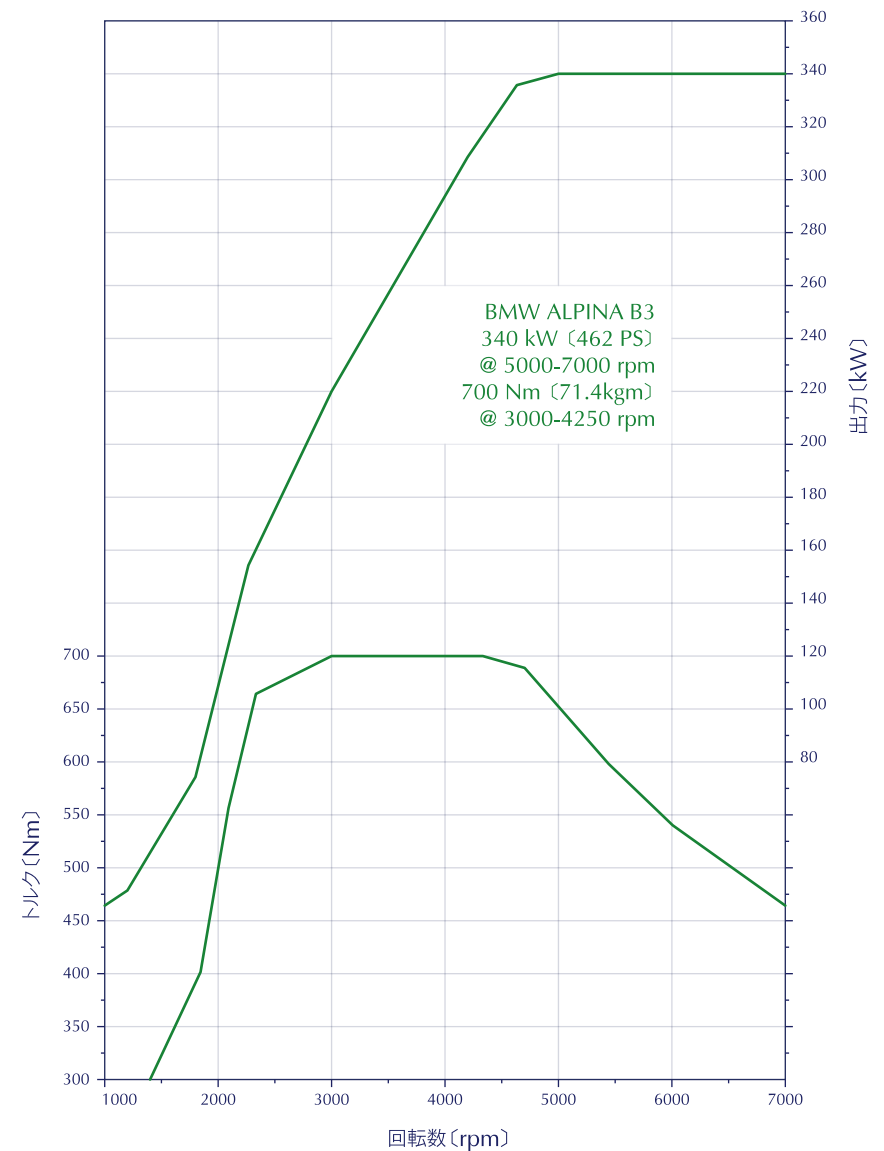
LEISTUNGS- UND DREHMOMENTDIAGRAMM BMW ALPINA B3 出力とトルク性能曲線
